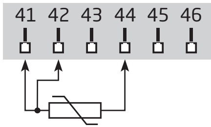
RTD 和线性电阻·3 线制
