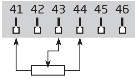
电位器
