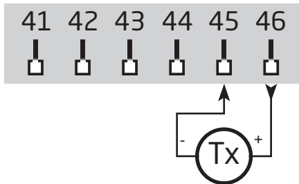
2 线制变送器
