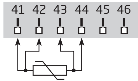
RTD 和线性电阻·4 线制
