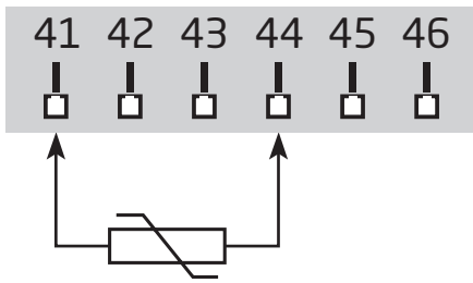
RTD 和线性电阻·2 线制
